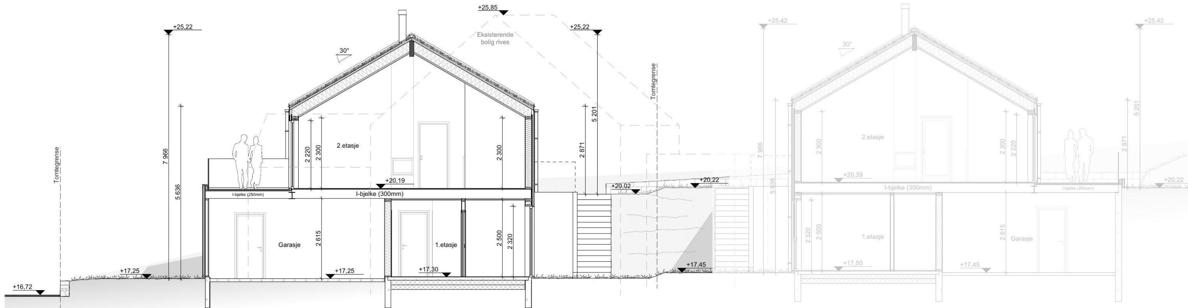
Snitt A-A bolig B
