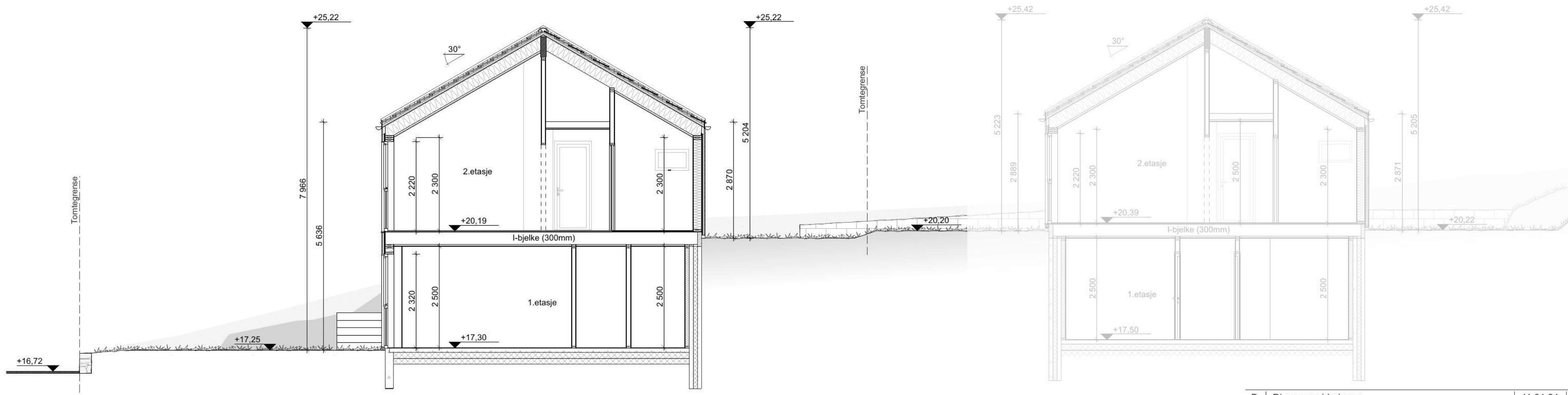
Snitt B-B bolig B
